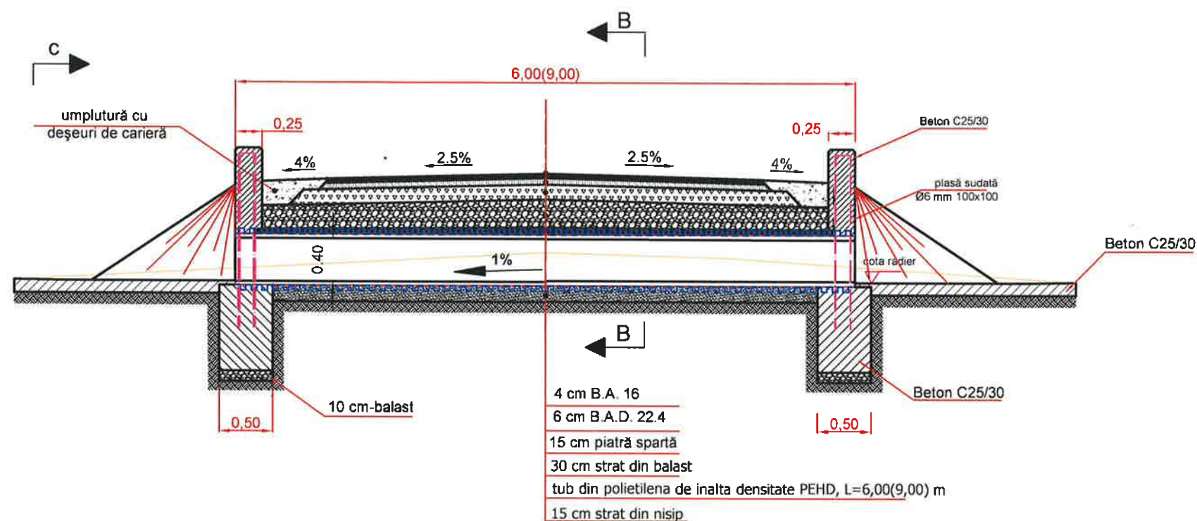
SECȚIUNE LONGITUDINALĂ PODEȚ: Ø 0.40 m; L = 6,00(9,00) m SECȚIUNEA A - A
